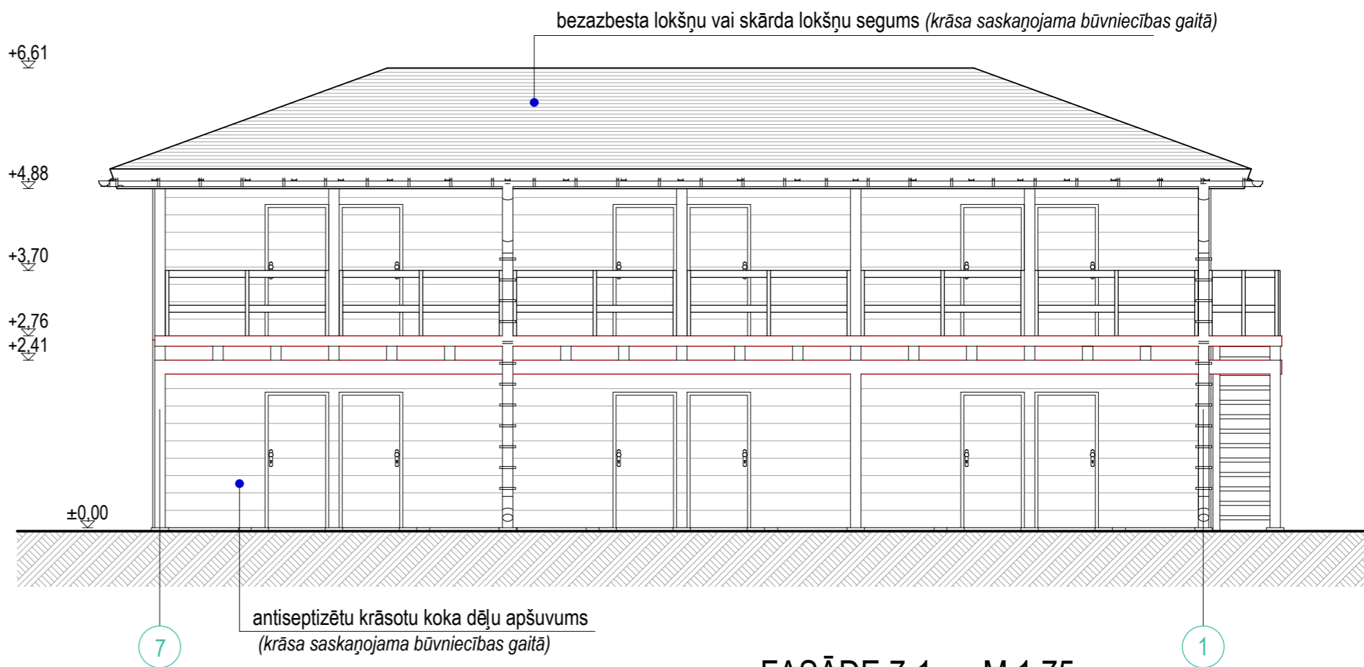
FASĀDE 7-1 M 1:75
